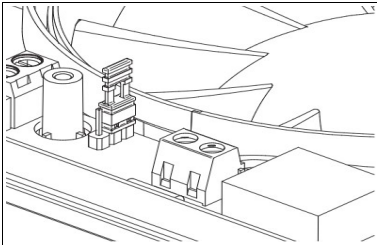
Ustawienie zworki – bieg niższy (domyślnie)
