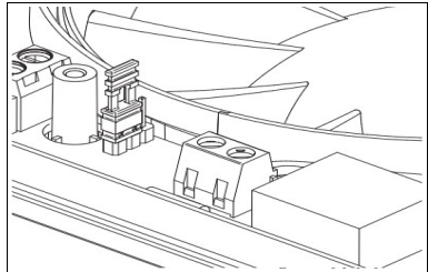
Ustawienie zworki – bieg wyższy
